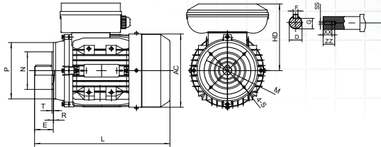
IM B14
